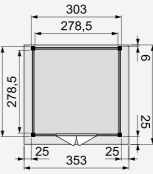
Zonder luifel
