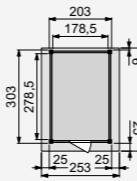
Zonder luifel
