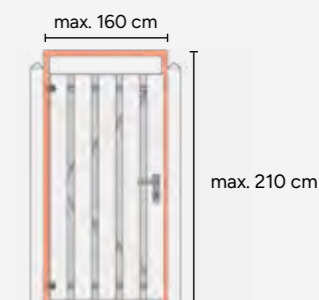
Tuindeurkozijn Universeel
