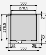
Zonder luifel
